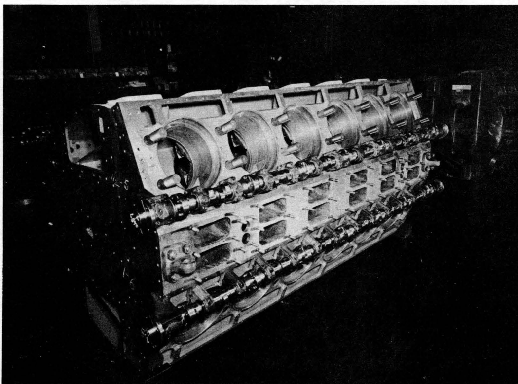
(Fig. 50) Model 567-A Crankcase
